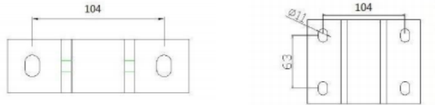
Figura 11 Posición del agujero del tornillo en los puntos fijos.
