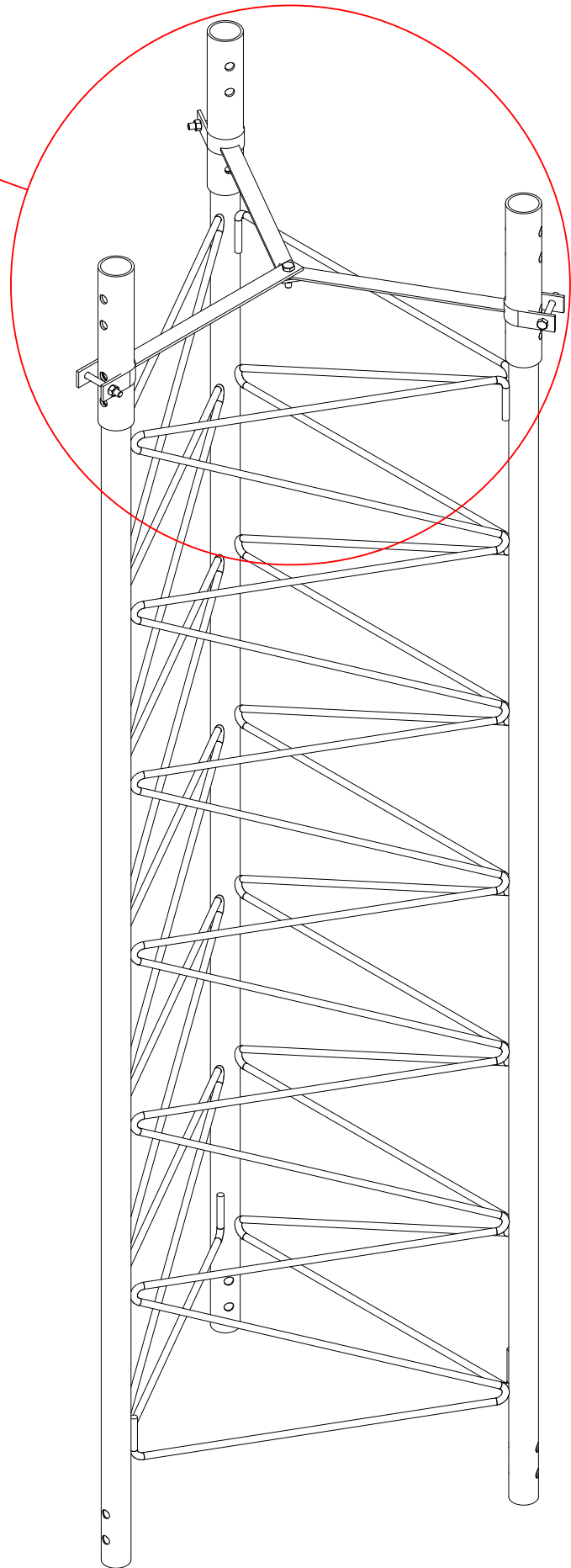
VISTA ISOMÉTRICA ENSAMBLAJE BRIDA 90 TRAMO STZ-90G
