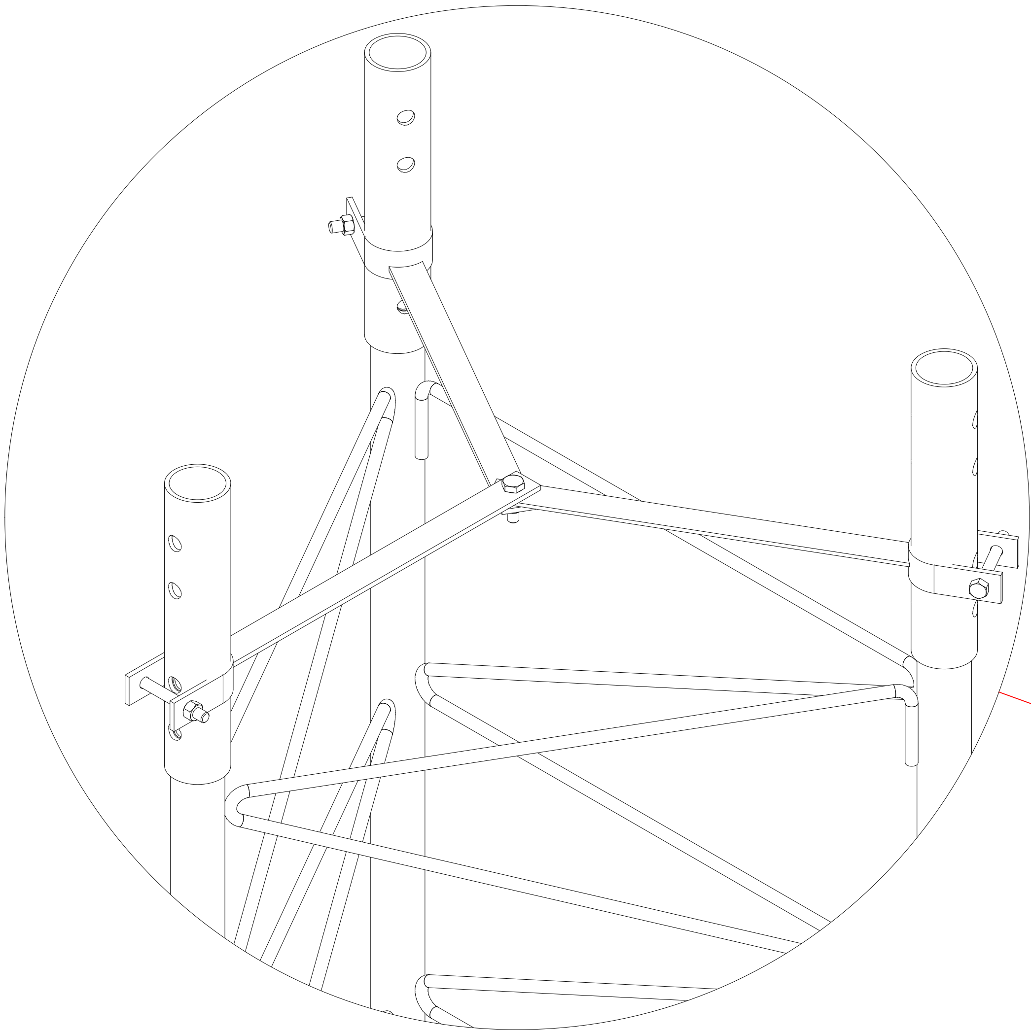
DETALLE BB ESCALA 1 : 4
