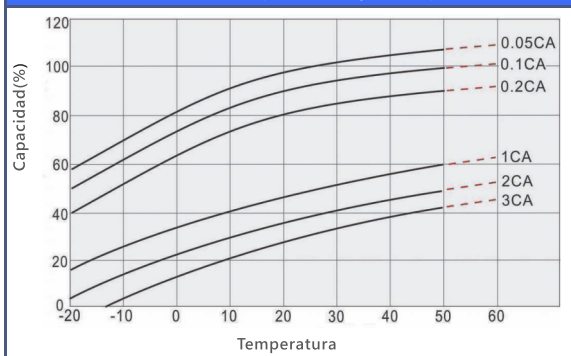
Relación entre la temperatura y la capacidad
