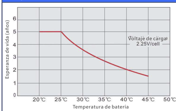
Temperatura vs Vida en flotación
