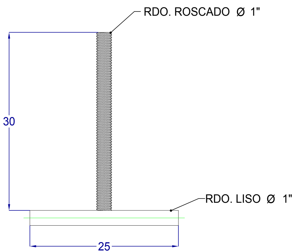
VISTA ELEVACIÓN
