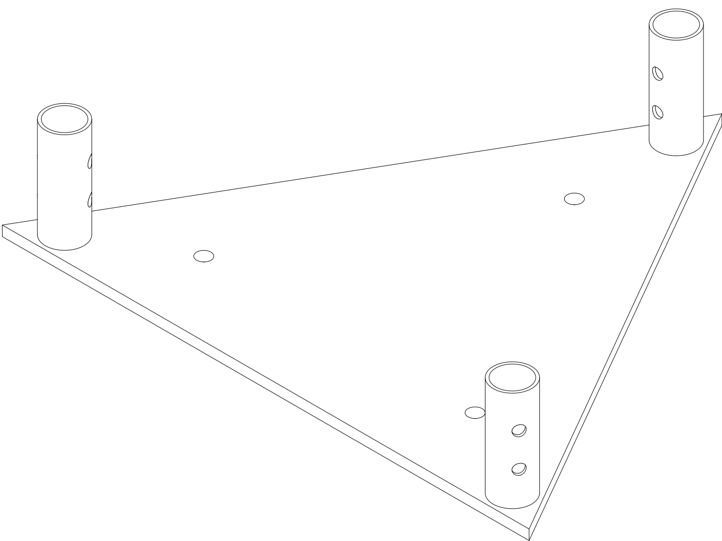
BASE SBA90G VISTA ISOMÉTRICA
