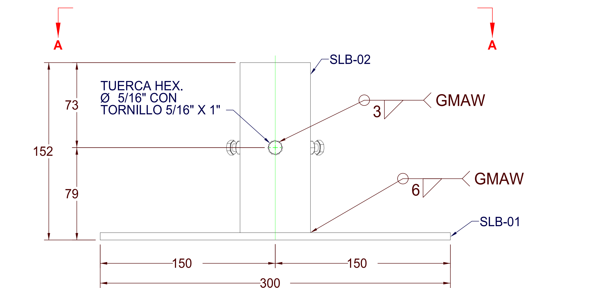
VISTA ELEVACION BASE CUADRADA SLM BAG
