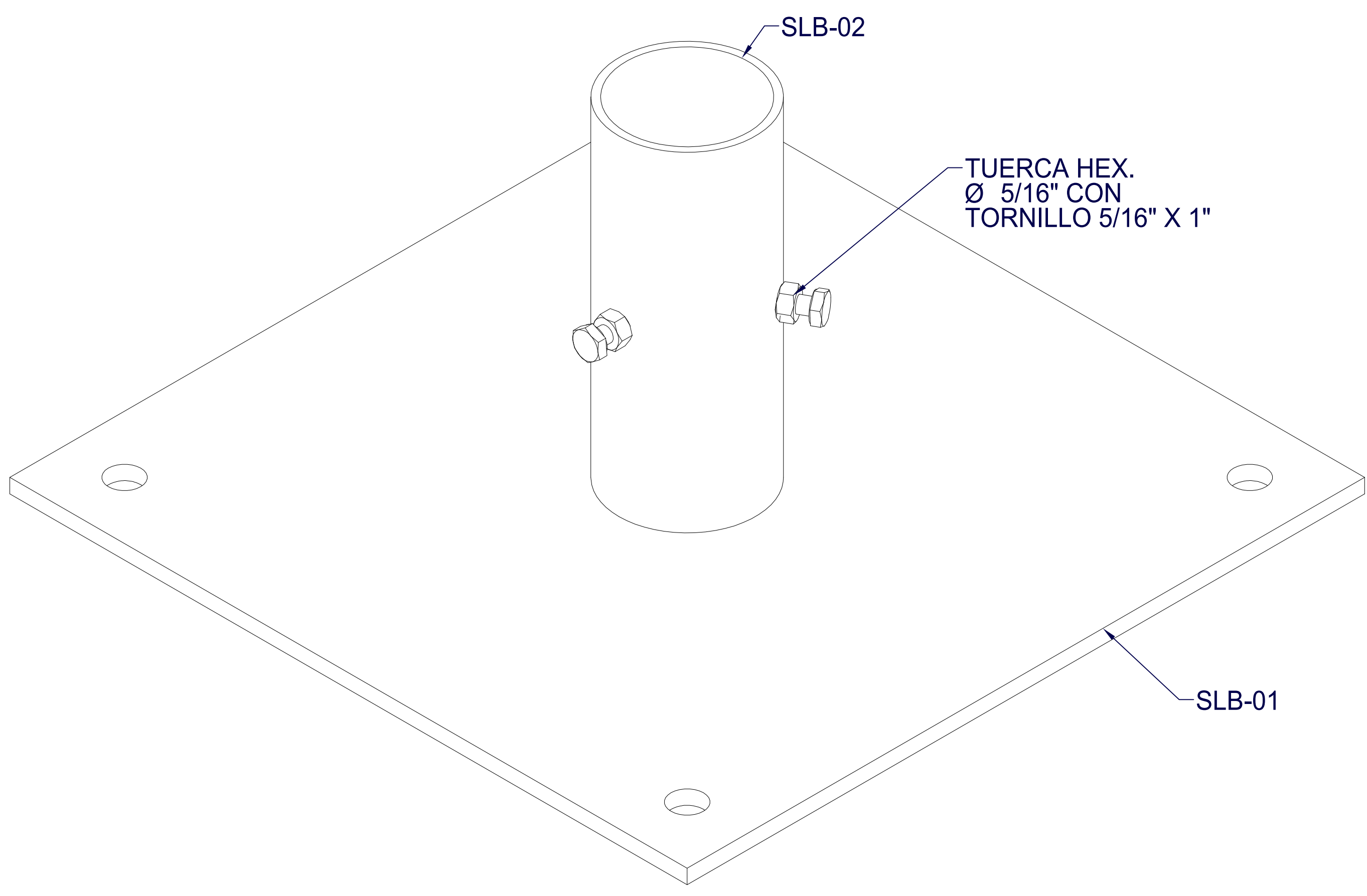
VISTA ISOMETRICA BASE CUADRADA SLMBAG
