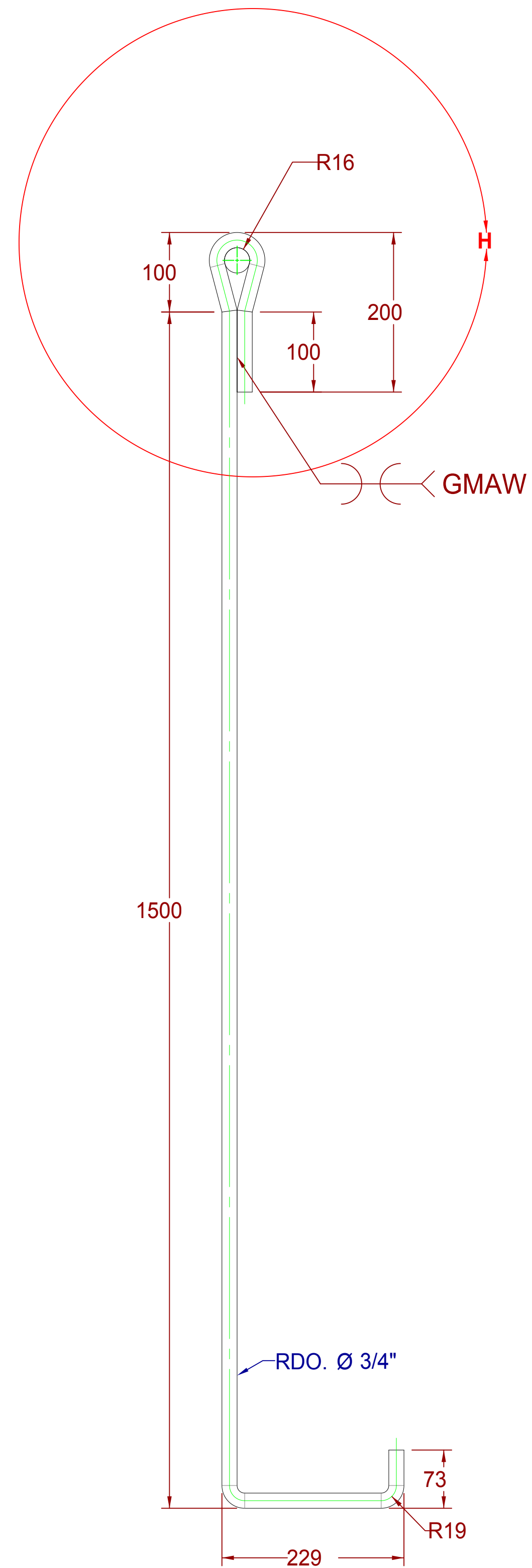
ANCLA SAZ-OL RDO. Ø 3/4"
