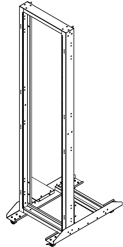
VISTA ISOMÉTRICA
