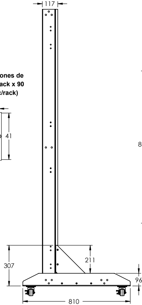
VISTA LATERAL
