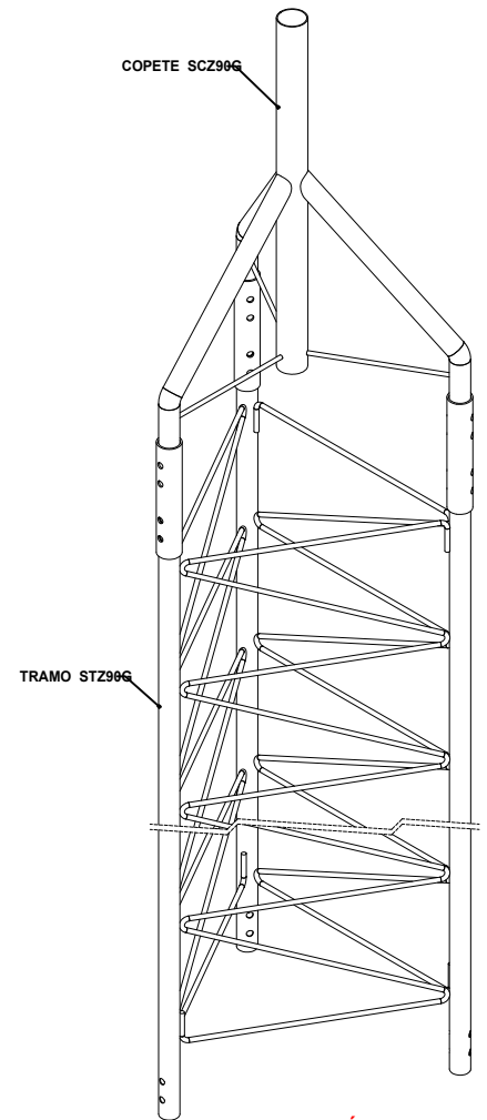
VISTA ISOMÉTRICA MONTAJE COPETE SCZ90G TRAMO STZ90G
