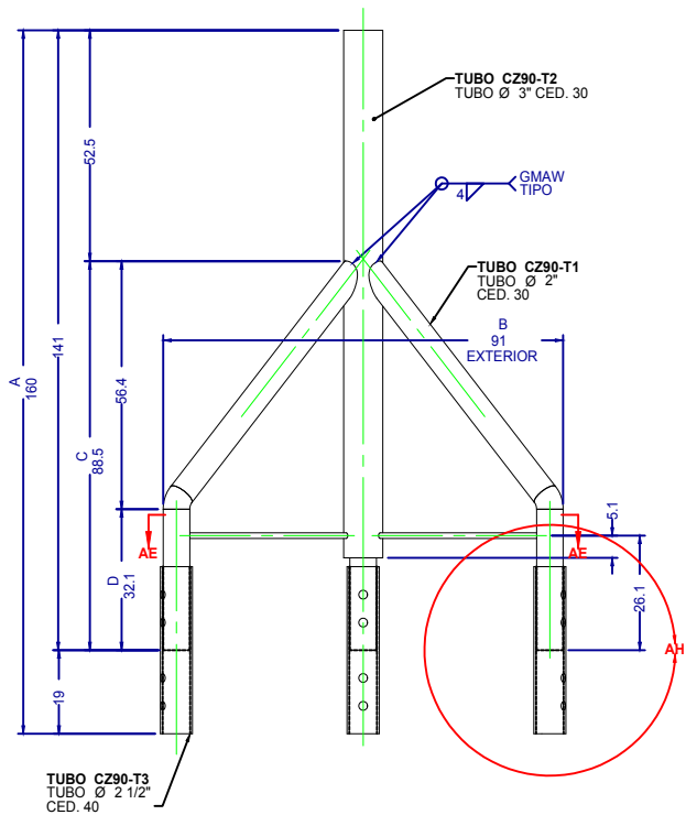
VISTA ELEVACIÓN COPETE SCZ90G
