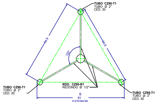
SECCIÓN AE-AE ESCALA 1:6
