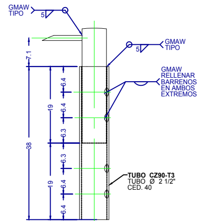
DETALLE AH ESCALA 1:3
