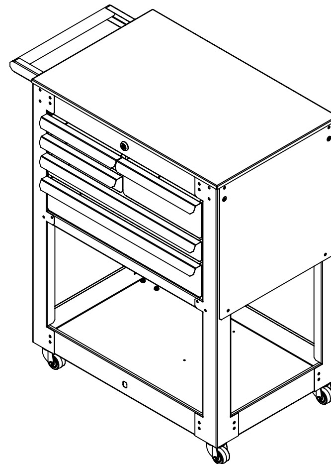
VISTA ISOMÉTRICA
