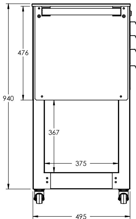
VISTA LATERAL
