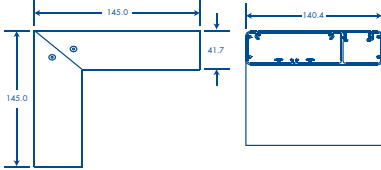
Esquinero interior
