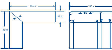
Sección L
