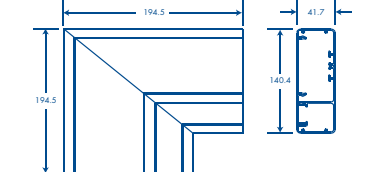
Sección T
