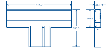
Sección T
