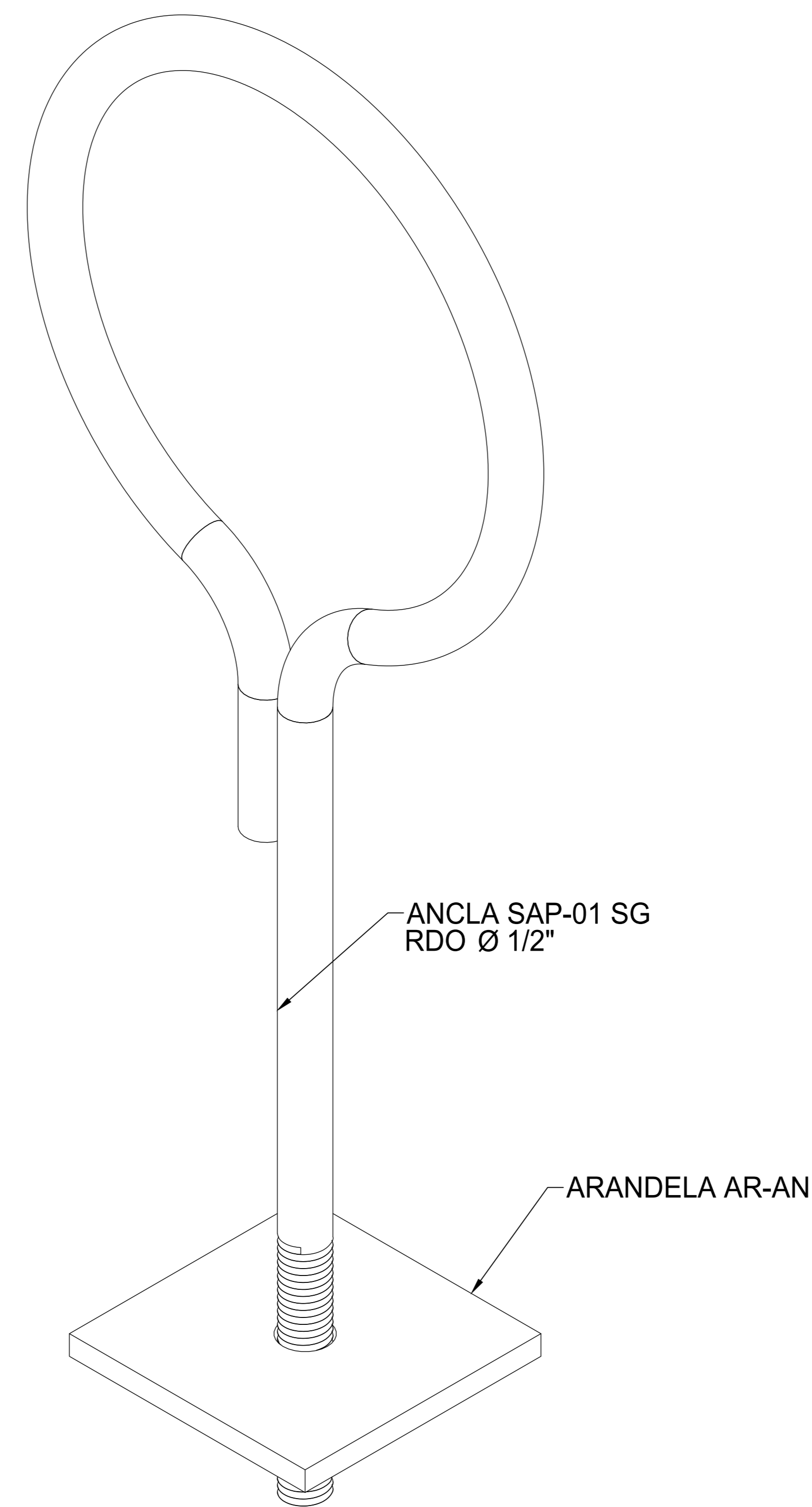
ANCLA SAP-01 SG VISTA ISOMÉTRICA
