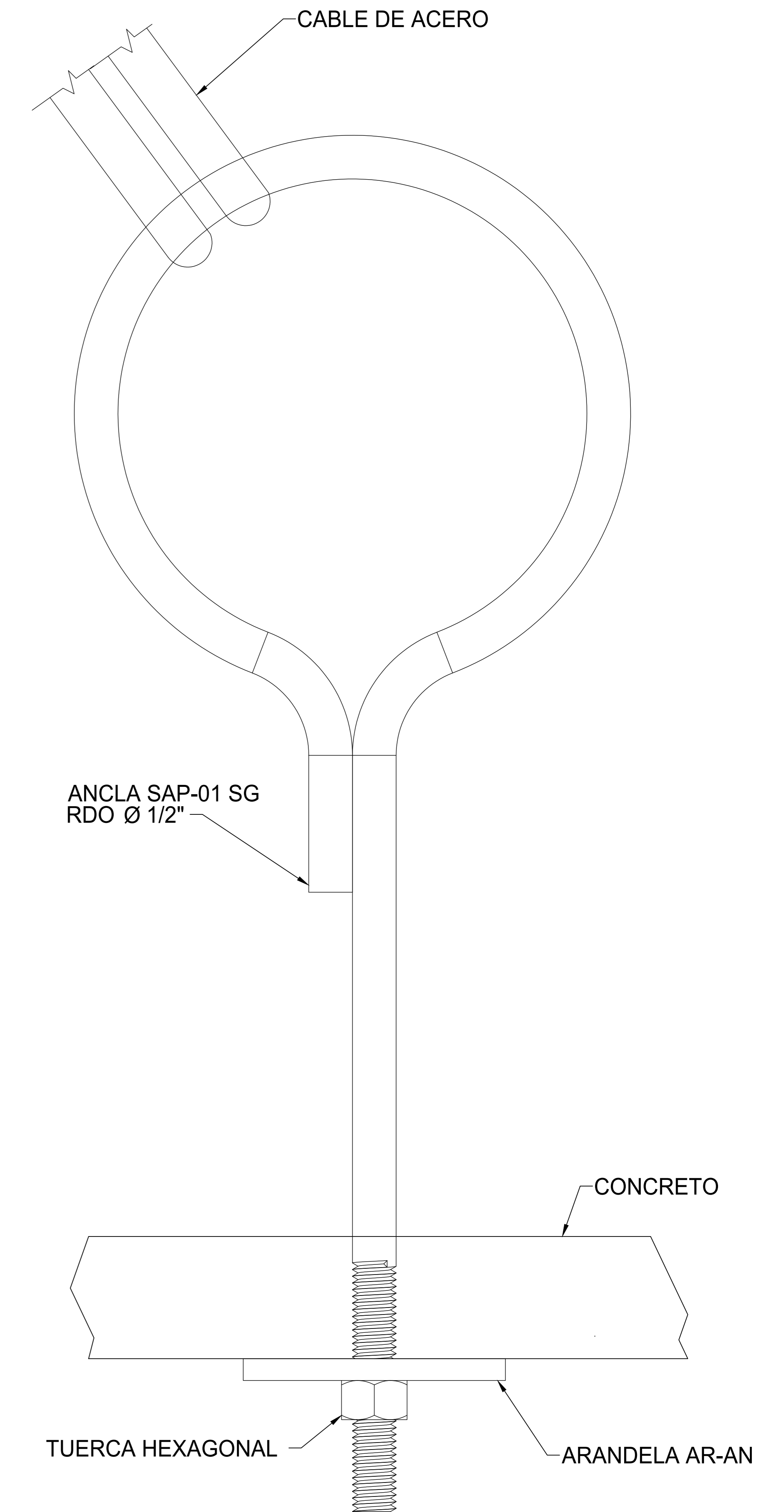
ANCLA SAP-01 SG VISTA MONTAJE
